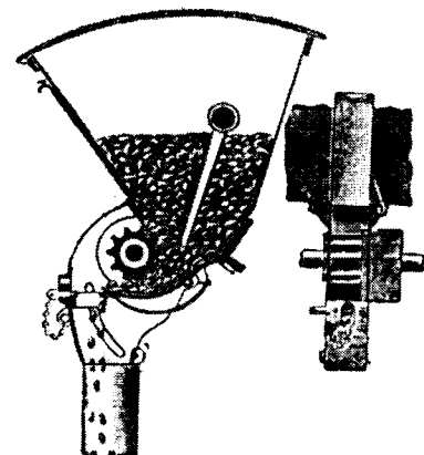
Шпультны высявальны прыбор Гузьера (2-я палова XIX ст.).
