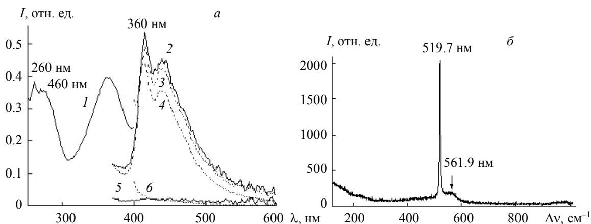
Рис. 5. Спектры люминесценции (а) образцов пленки ZnO+0.9%Sc 2 O 3 на кремнии (2—4) и подложек кремния (5, 6) при \lambda_{\text{возб}} = 260 (2), 280 (3, 5) и 340 нм (4, 6), I — спектр возбуждения люминесценции образца пленки на кремнии; \lambda_{\text{рег}} = 460 нм; б — КР-спектр тонких пленок на кремниевой подложке
