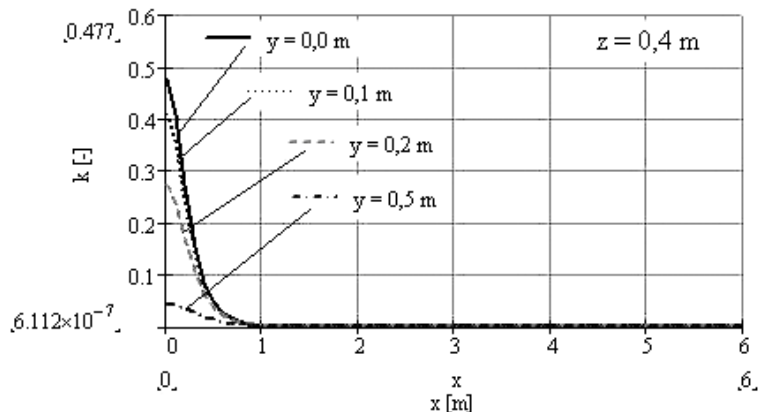
Rys. 4. Zmiana wartości współczynnika k(x) dla punktu gleby A(0,y,z) dla wybranych wartości współrzędnej y Fig. 4. Changes in the values of the coordinate k(x) for the soil point A(0, y, z) , for the selected values of the coordinate y
