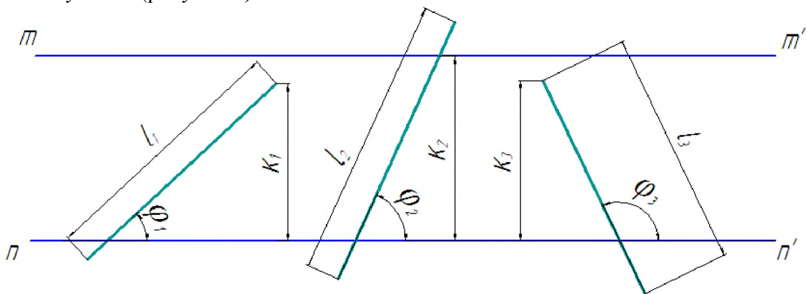
Рисунок 3. – Схема расположения остатков стеблей относительно ножей катка
