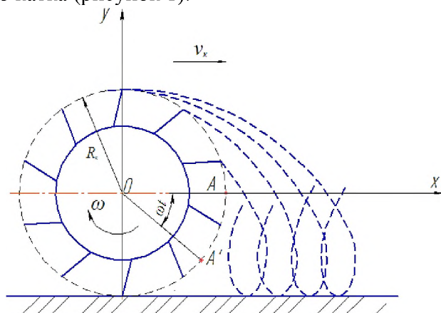
Рисунок 1. – Траектории движения точки A лезвий ножей спирально-ножевидного катка
