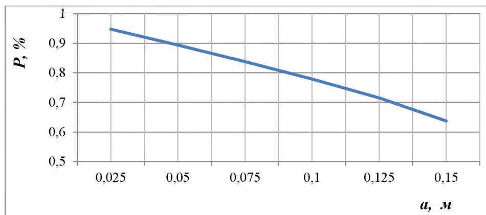
Рисунок 5. – Зависимость вероятности измельчения растительных остатков от шага расстановки ножей спирально-ножевидного катка
