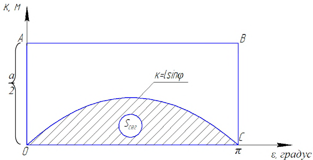
Рисунок 2. – Схема прямоугольника OABC и сегмента S_{сез} , определяющих вероятность попадания ножа на растительный остаток
