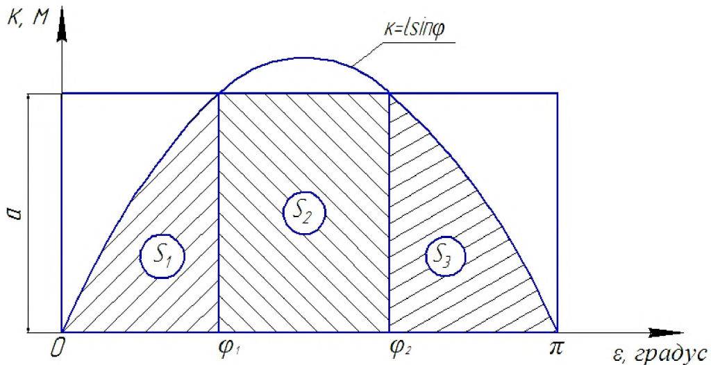
Рисунок 4. – Схема для определения вероятности перерезания остатка стебля одним или двумя ножами катка, установленными с шагом a
